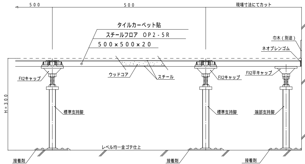
断面図 S = 1 : 5
